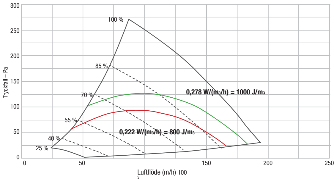
Flödesdiagram
